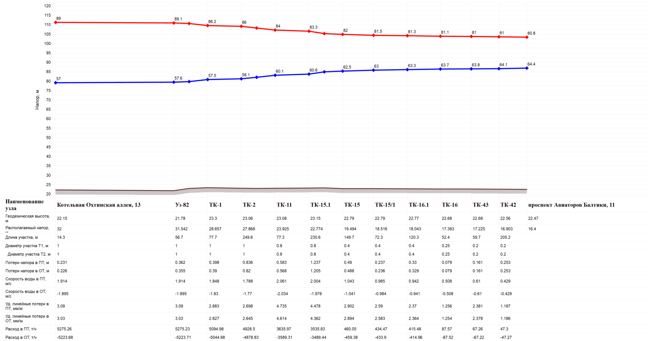
Рисунок 15. Пьезометрический график от котельной ООО «Петербургтеплоэнерго» до проспект Авиаторов Балтики, 11
