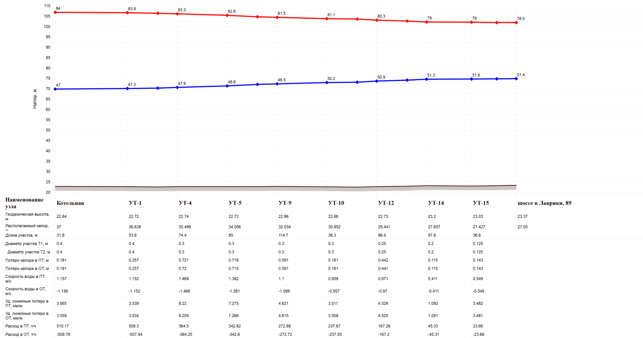
Рисунок 21. Пьезометрический график от котельной ООО «ЖилКомТеплоЭнерго»
