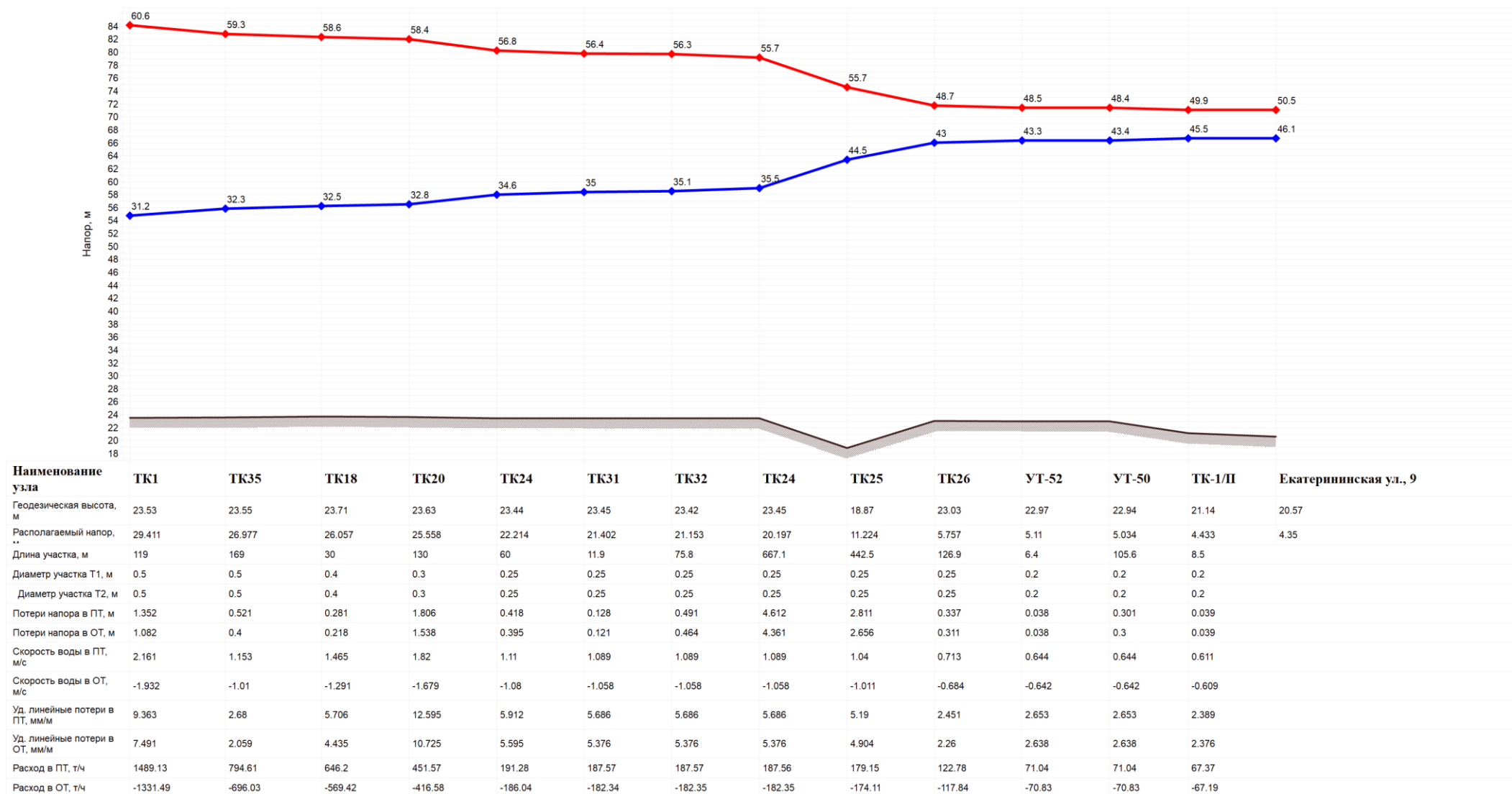
Рисунок 24. Пьезометрический график от котельной ООО «ГАЗКОМПЛЕКТ» ул. Екатерининская 32, стр. 1 до ул. Екатерининская, д. 9
