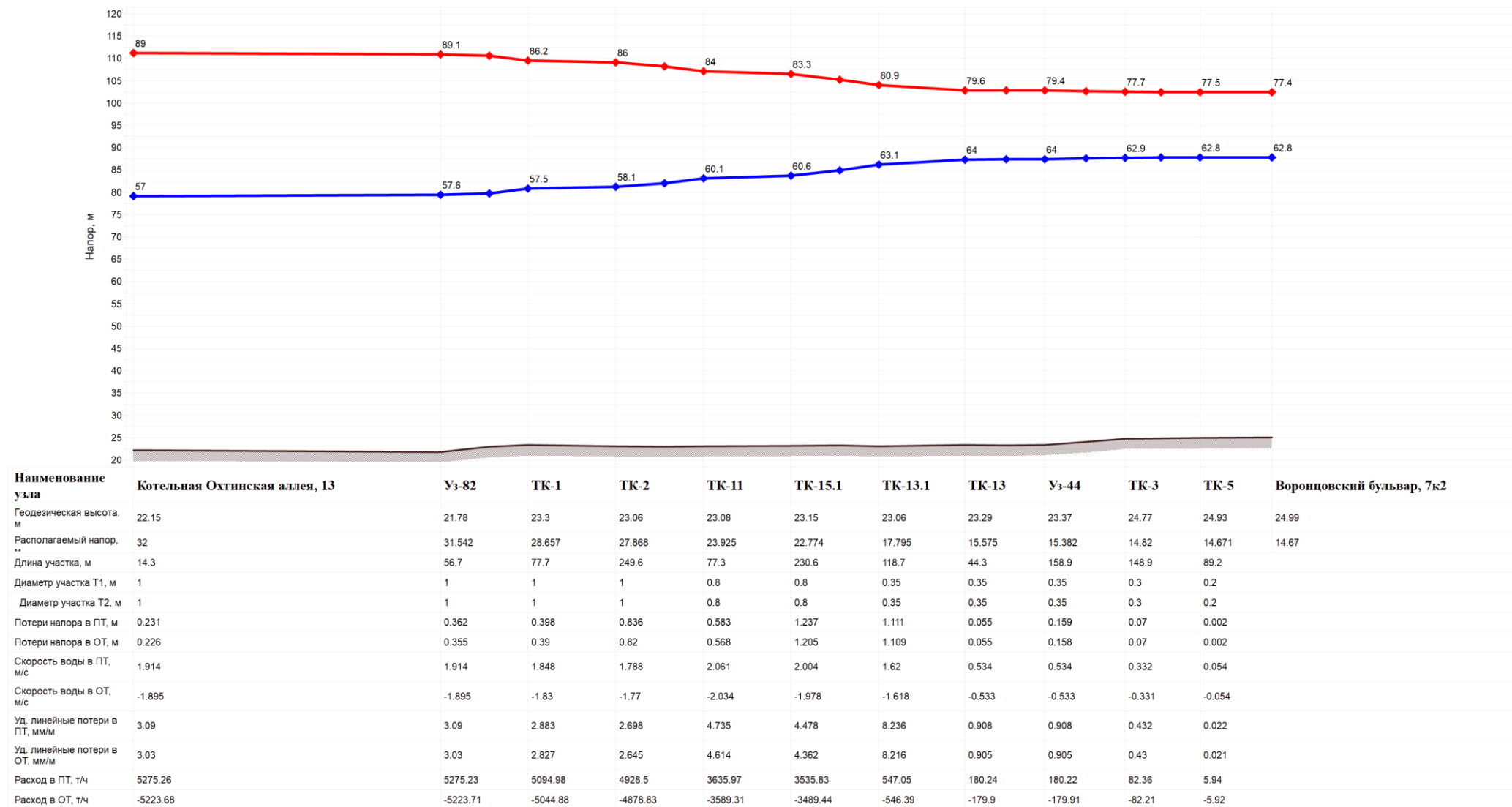
Рисунок 16. Пьезометрический график от котельной ООО «Петербургтеплоэнерго» до Воронцовский бульвар, 7к2
