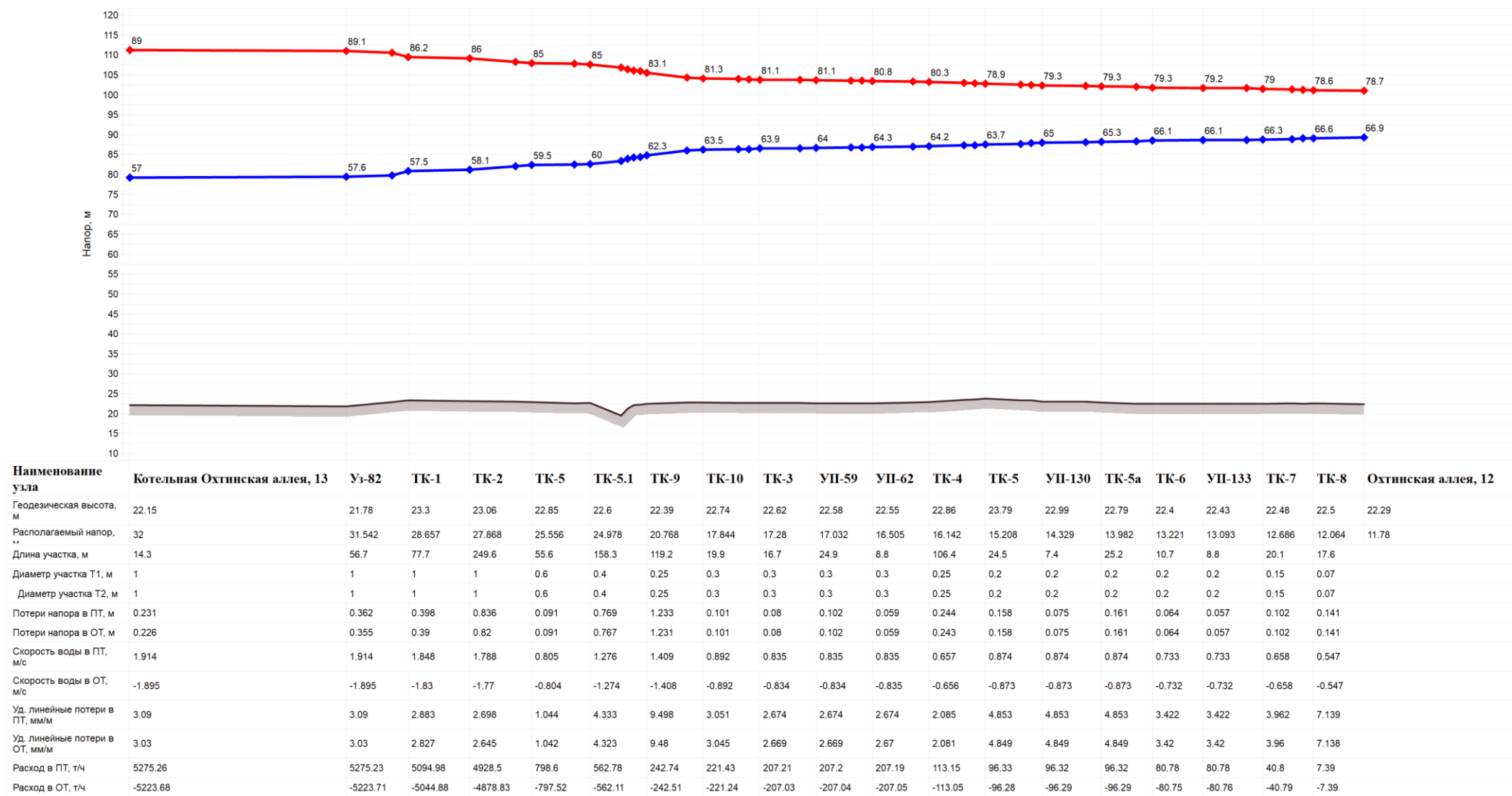
Рисунок 18. Пьезометрический график от котельной ООО «Петербургтеплоэнерго» до Охтинской аллеи 12
