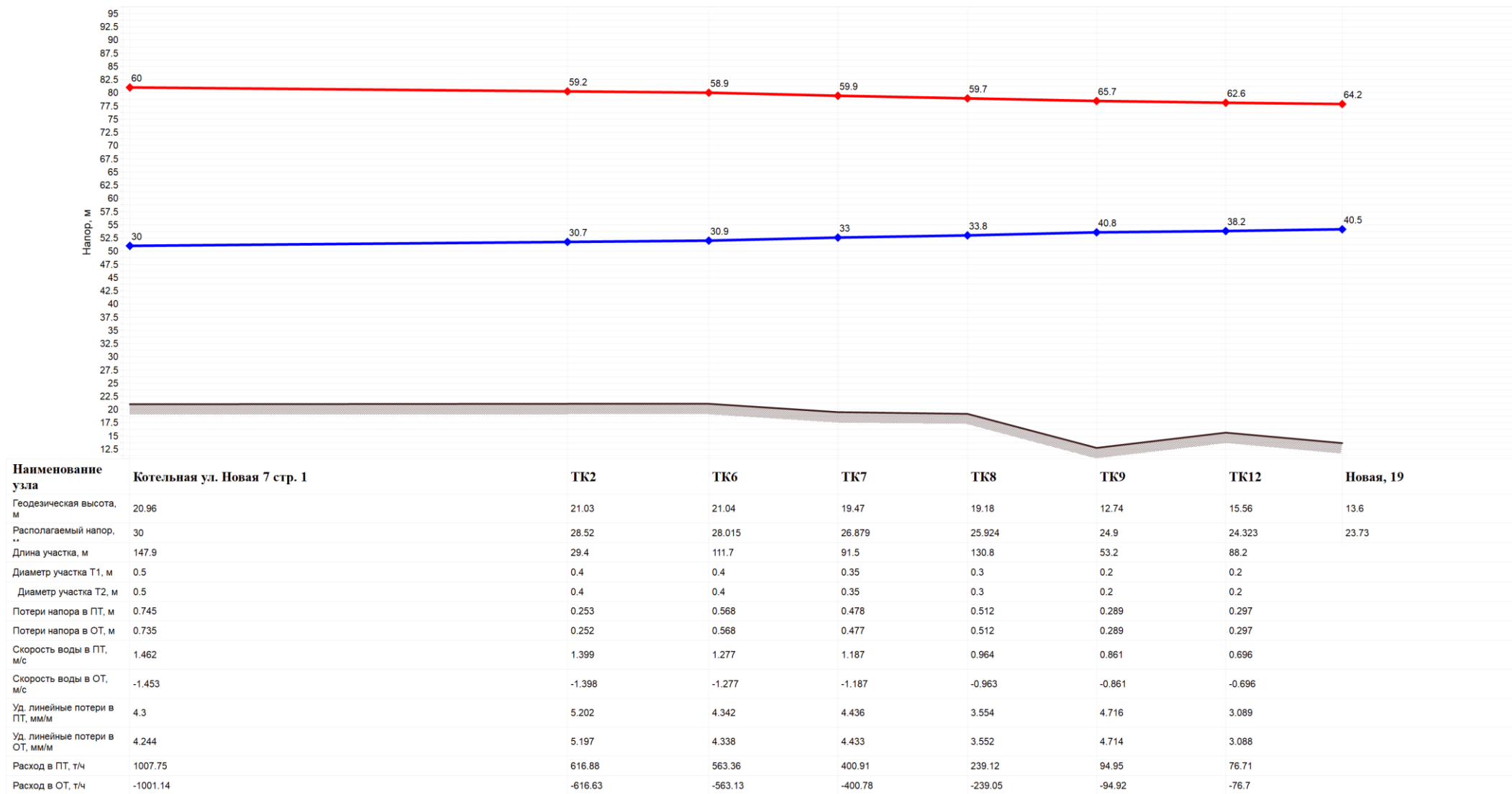
Рисунок 23. Пьезометрический график от котельной ООО «ГАЗКОМПЛЕКТ» ул. Новая, д. 7
