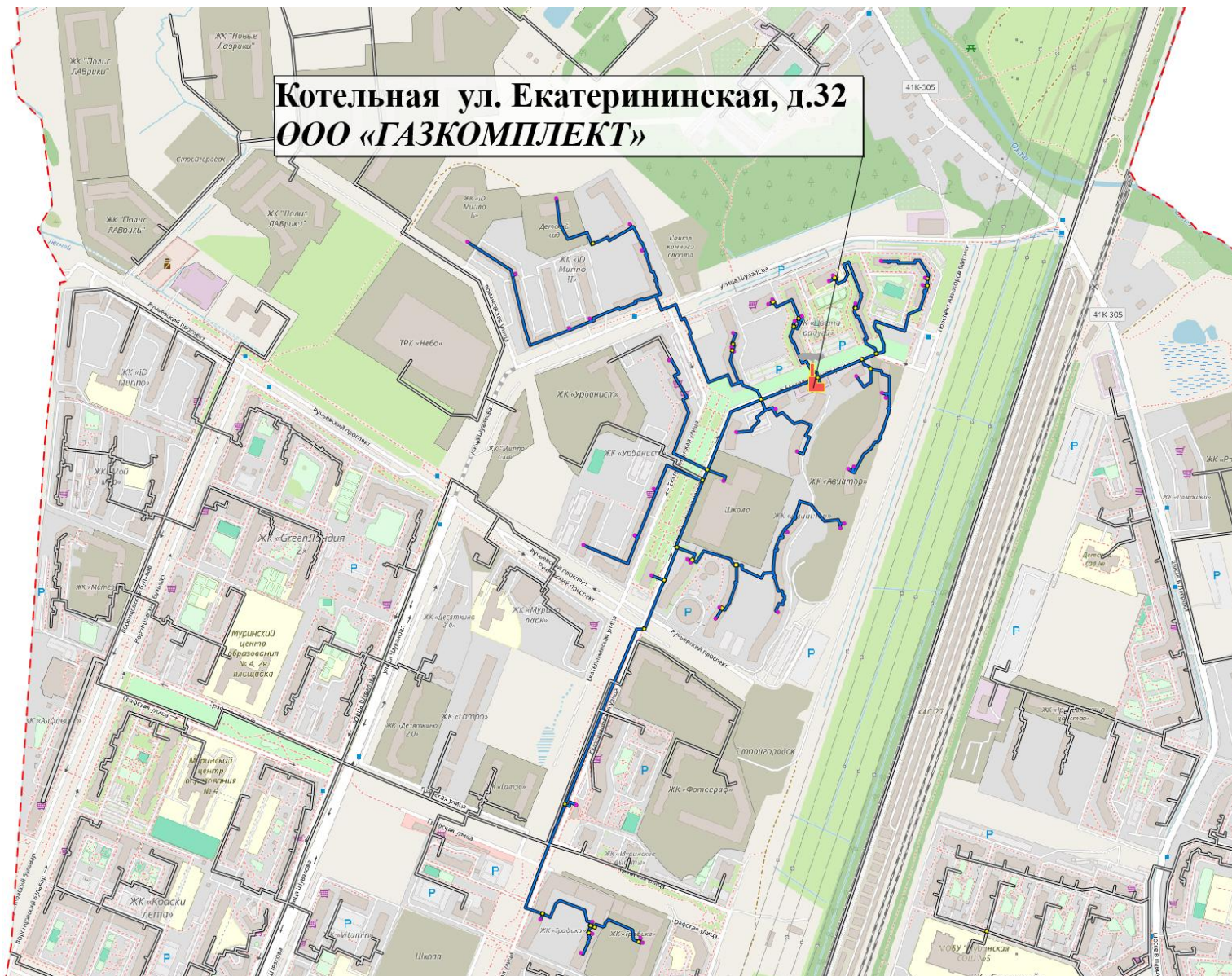
Рисунок 10. Схема тепловых сетей котельной ООО «ГАЗКОМПЛЕКТ» ул. Екатерининская, д. 32, стр. 1
