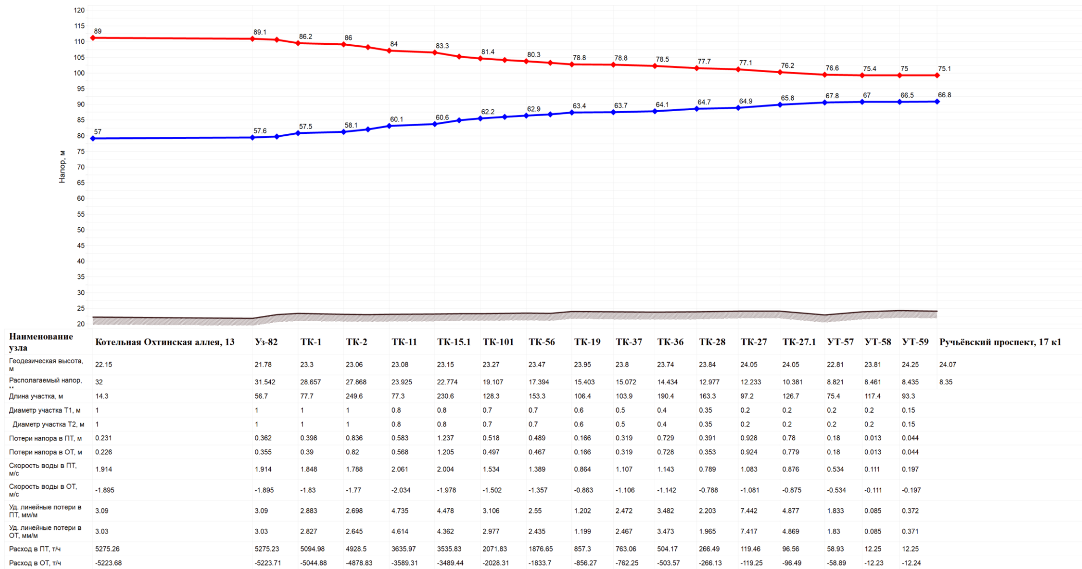
Рисунок 19. Пьезометрический график от котельной ООО «Петербургтеплоэнерго» до Ручьевский проспект 17 к 1
