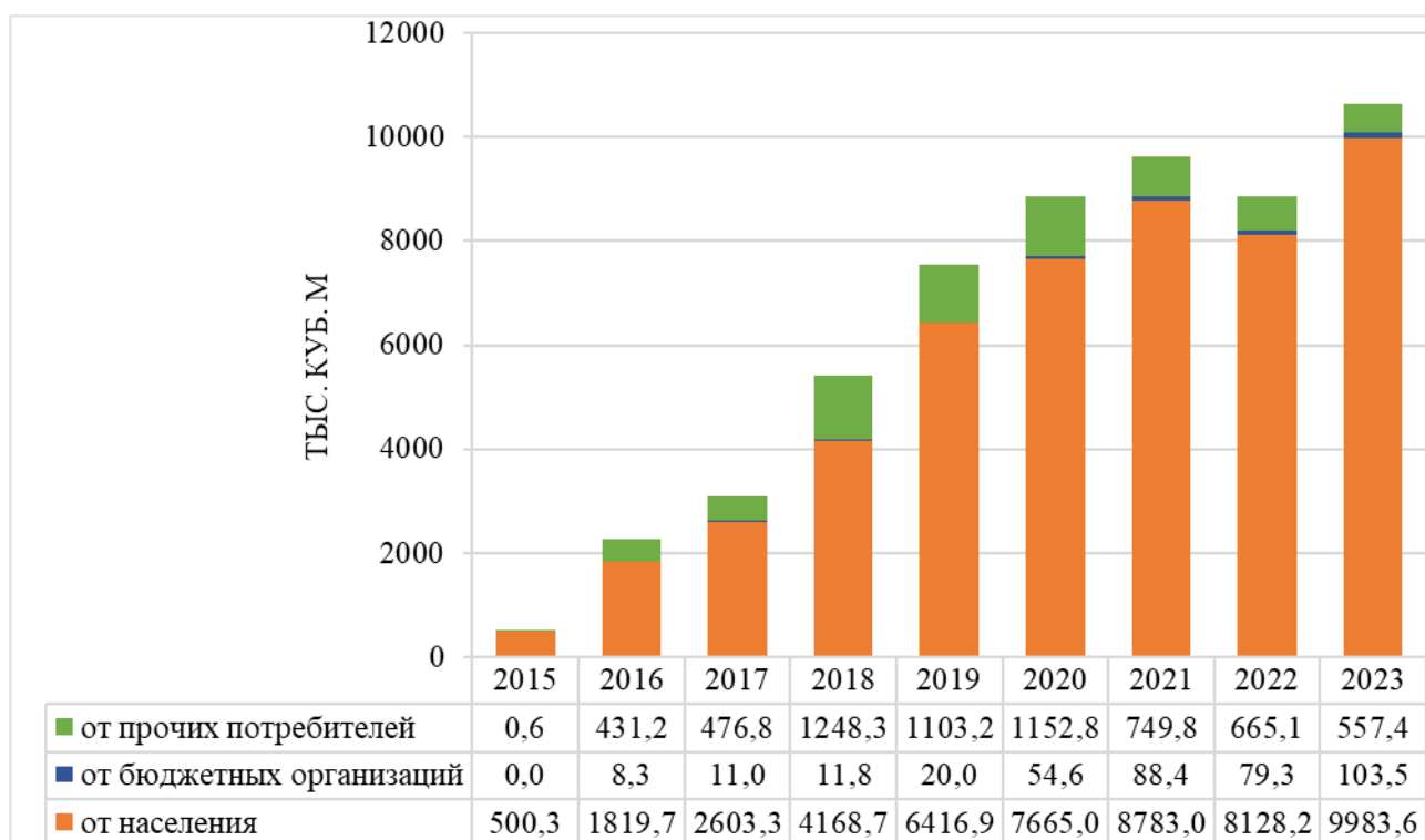
Рисунок 2.28. Ретроспективный баланс поступления сточных вод Муринского городского поселения за 2015 — 2023 гг.
