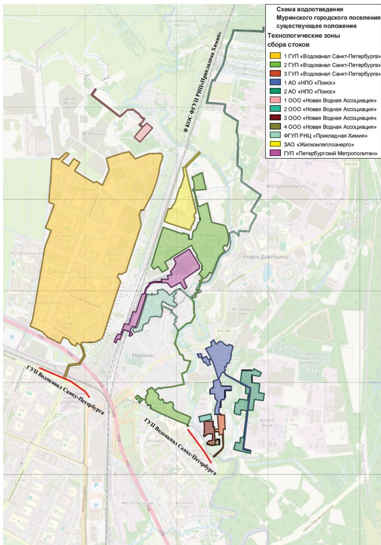
Рисунок 2.9. Технологические зоны водоотведения (зоны сбора стоков) Муринского городского поселения
