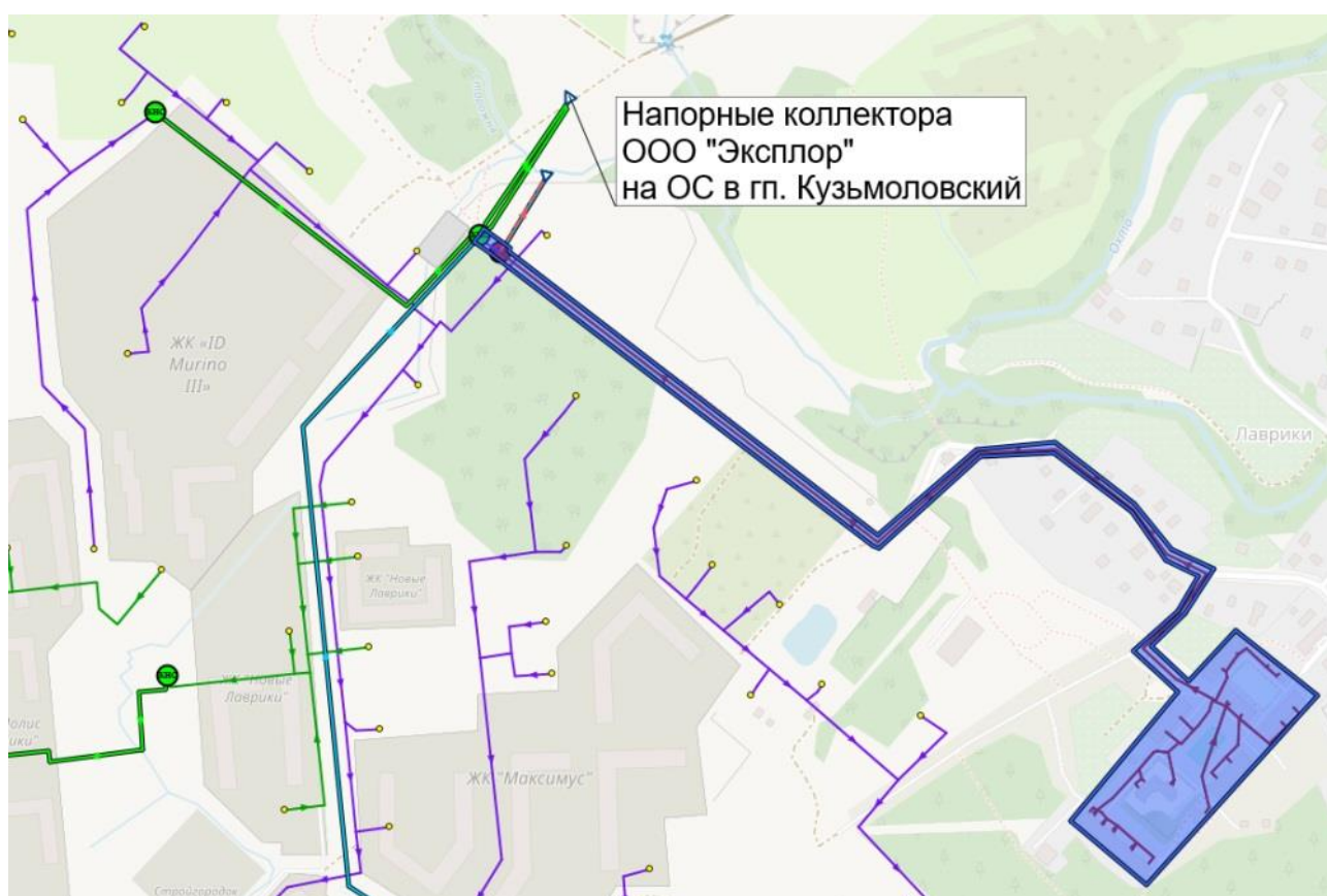
Рисунок 2.32. Схема подключения системы водоотведения д. Лаврики к очистным сооружениям
