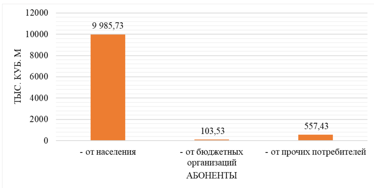
Рисунок 2.25. Структура отведенных стоков по Муринскому городскому поселению за 2023 год
