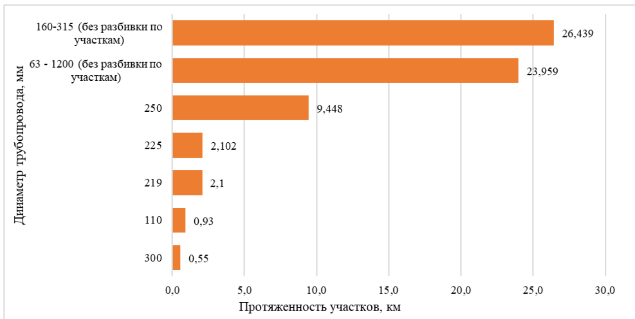
Рисунок 2.11. Долевое распределение по диаметрам трубопроводов сетей водоотведения Муринского городского поселения
