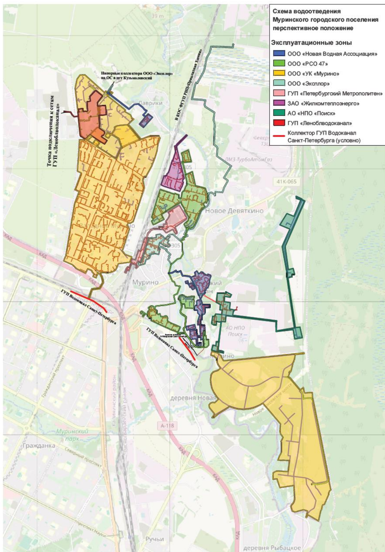
Рисунок 2.36. Перспективное расположение эксплуатационных зон РСО Муринского городского поселения –Сценарий 3 (общий вид)
