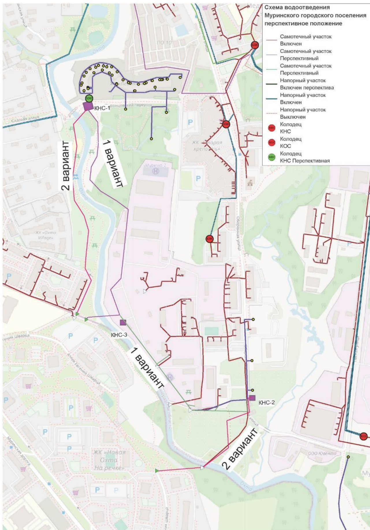
Рисунок 2.30. Схема подключения жилых домов по ул. Оборонная к сетям ООО «PCO 47 (варианты 1 и 2)
