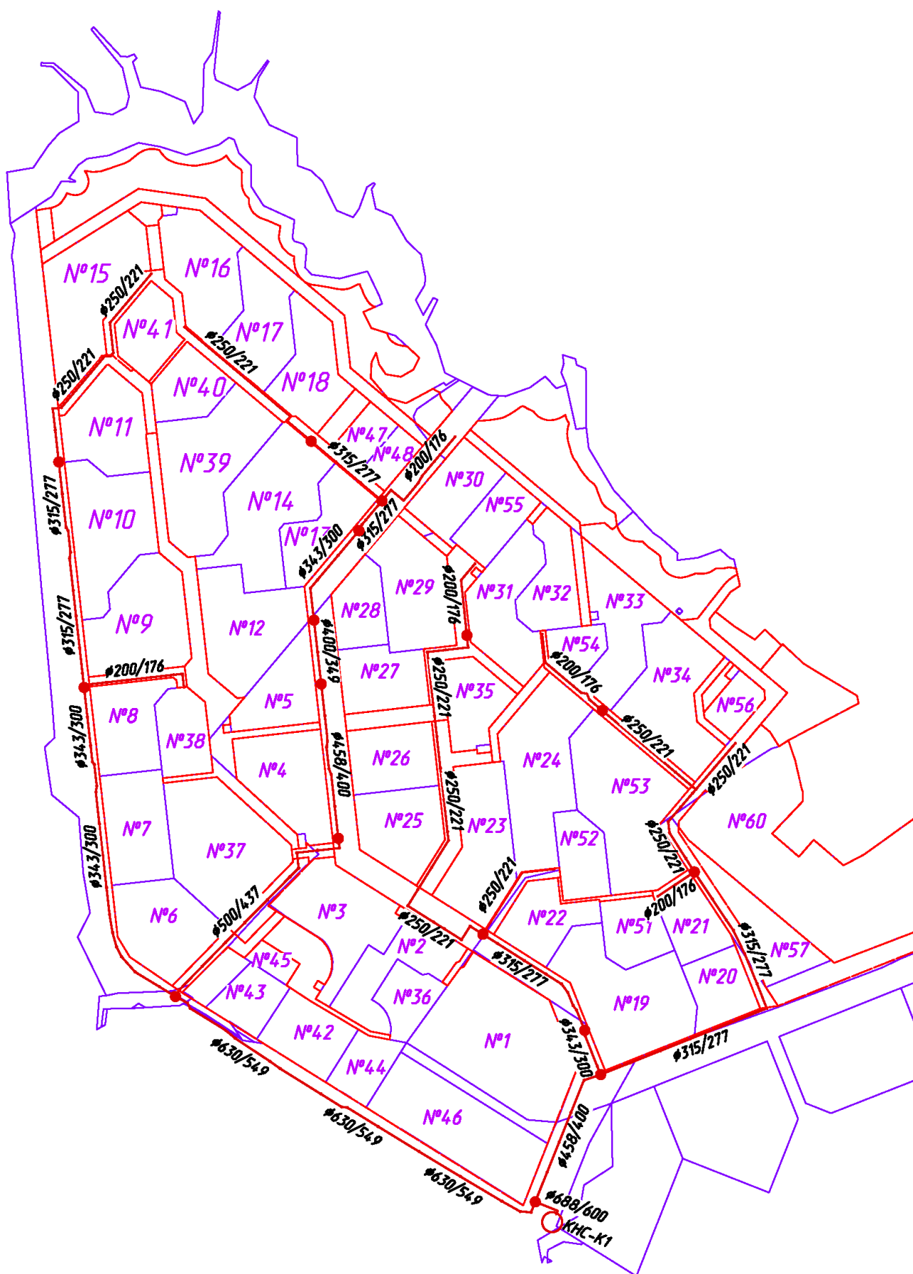
Рисунок 1.34. Схема сетей водоотведения ООО «УК «Мурино» (согласно ППТ № 200)
