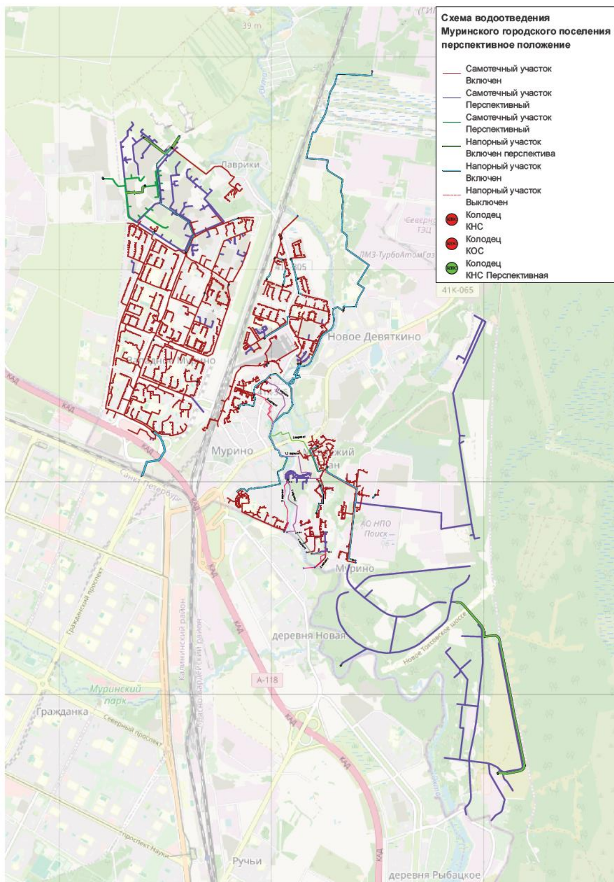
Рисунок 2.33. Перспективная схема сетей водоотведения Муринского городского поселения (общий вид)
