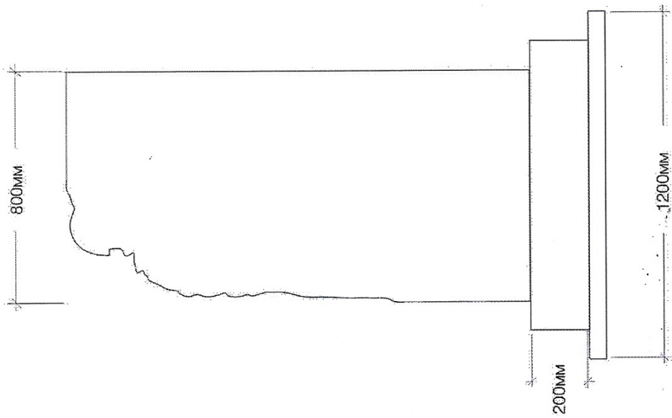
вид спереди
