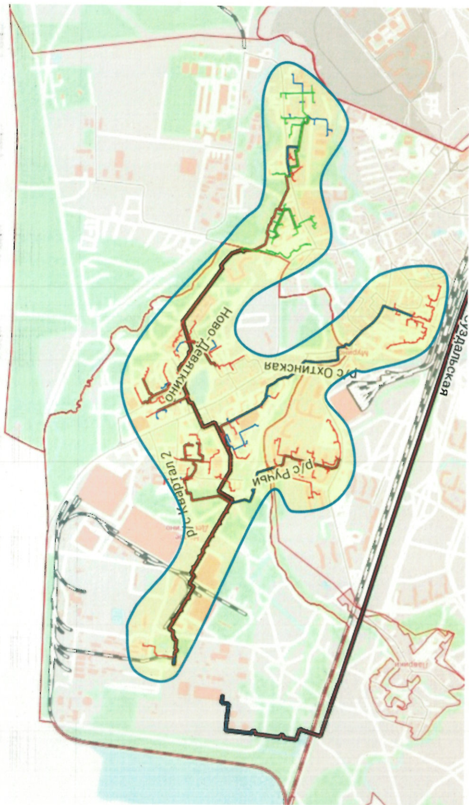
Общий вид зоны гидравлических испытаний на прочность и плотность т/м Ново-Девяткино с тепловыми вводами на территории дер. Новое Девяткино и гор. Мырино
