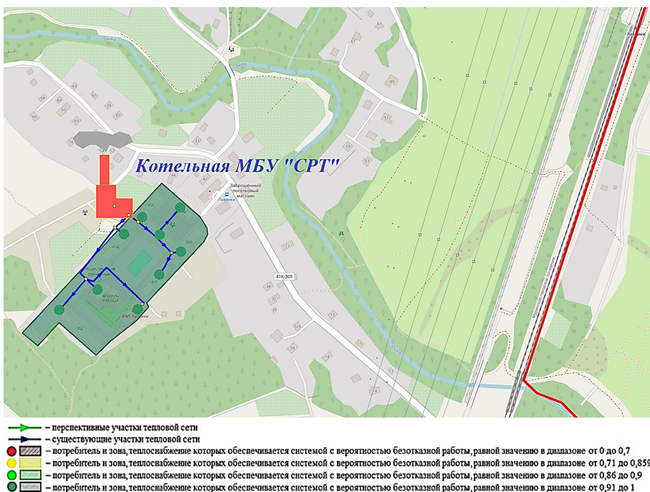
Рисунок 17. Зона, характеризующая надежность теплоснабжения потребителей котельной МБУ «СРТ» на период до 2030 года в границах муниципального образования «Муринское городское поселение»
