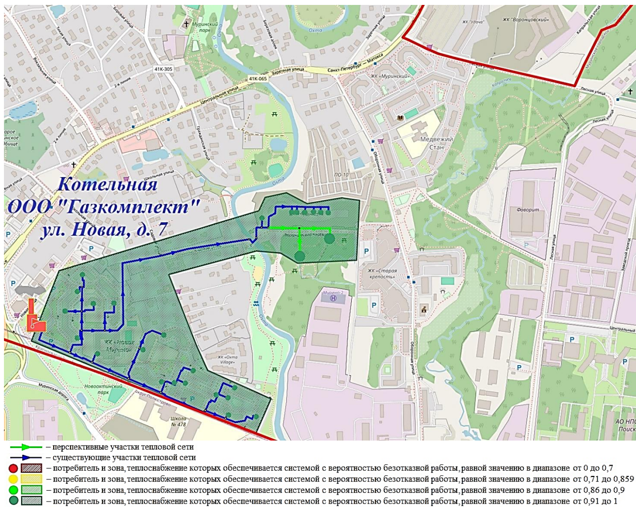
Рисунок 9. Зона, характеризующая надежность теплоснабжения потребителей котельной ООО «Газкомплект» по адресу ул. Новая, д. 7 на период до 2030 года в границах муниципального образования «Мурманское городское поселение»
