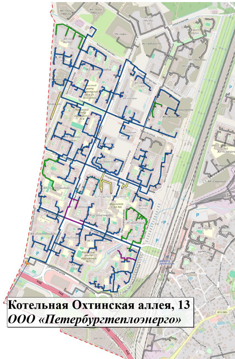
Рисунок 5. Схема тепловых сетей котельной ООО «Петербургтеплоэнерго»
